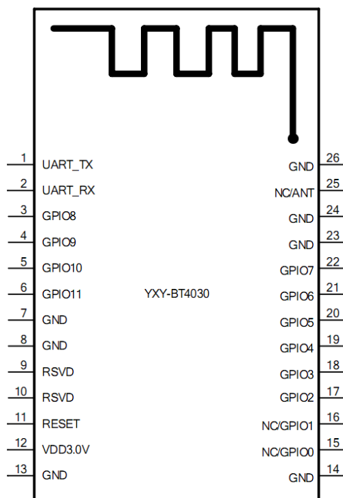
图 2. PIN 脚分布
